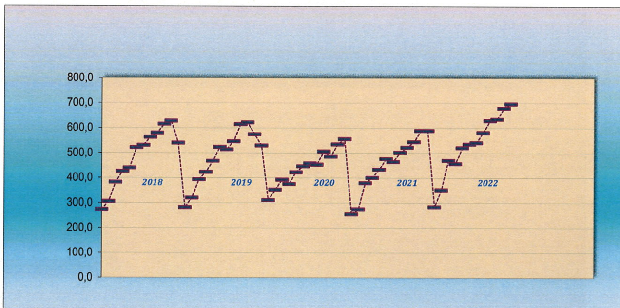
Graf č. 2 : Vývoj stavebnej produkcie (podniková metóda) v rokoch 2018-2022 v mil. Eur
