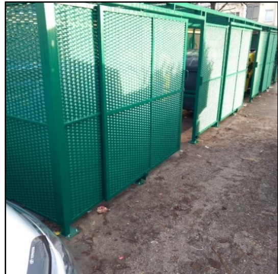
Obr. 6 Kontajnerovisko Hollého
