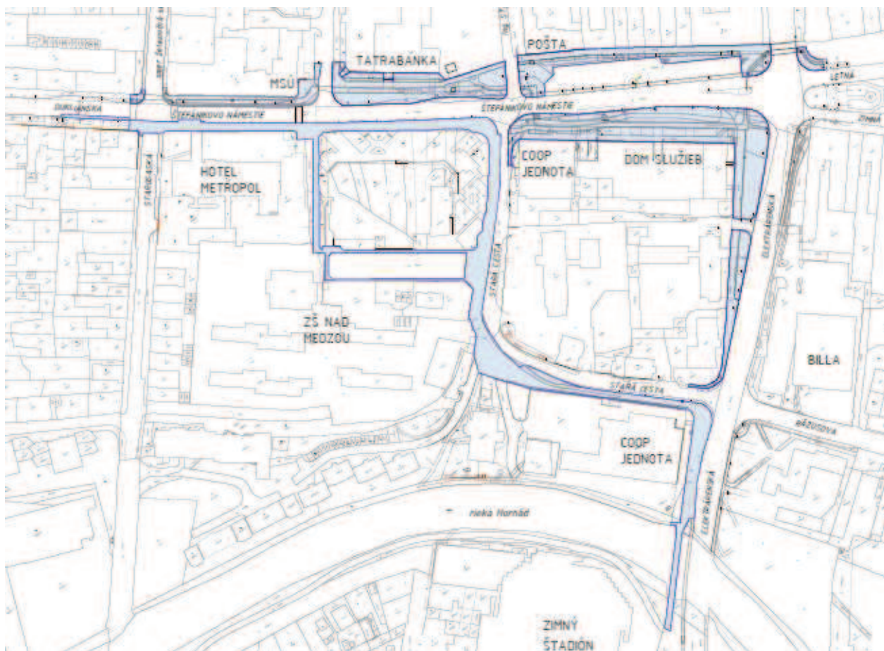
Obrázok č. 27 Prestavba chodníkov a spevnených plôch s vytvorením cyklistických trás v centre mesta Spišská Nová Ves
