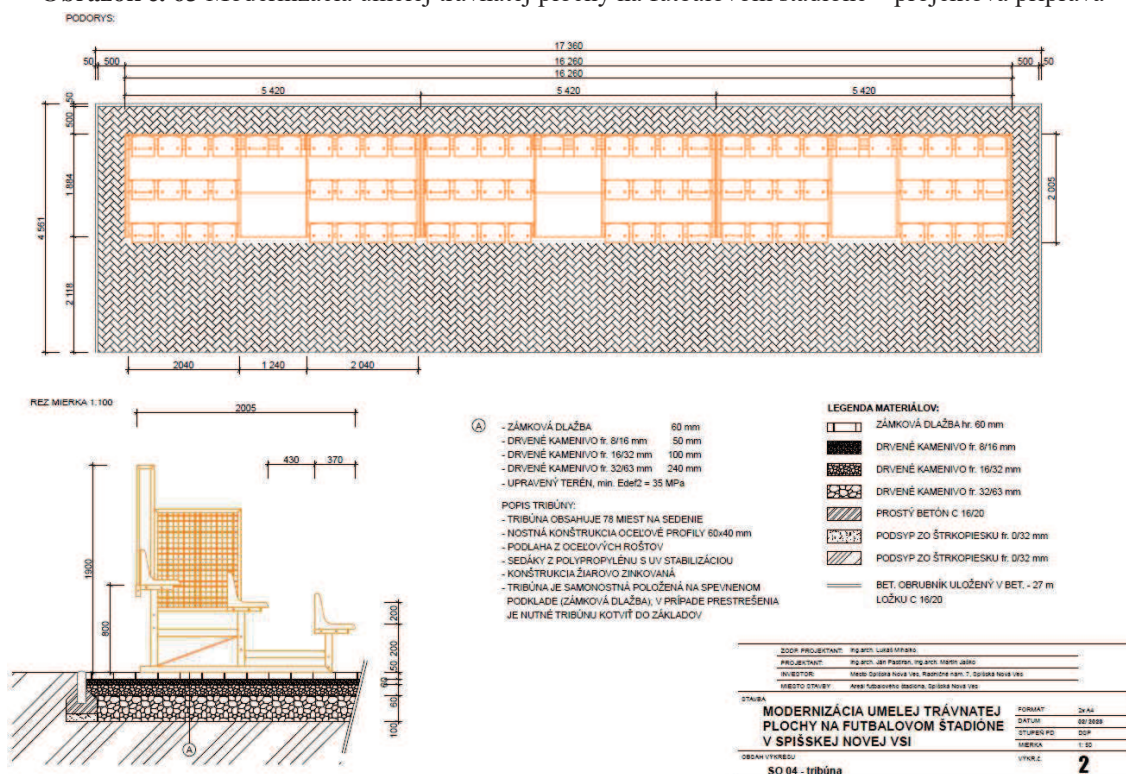
Obrázok č. 63 Modernizácia umelej trávnej plochy na futbalovom štadióne – projektová príprava
