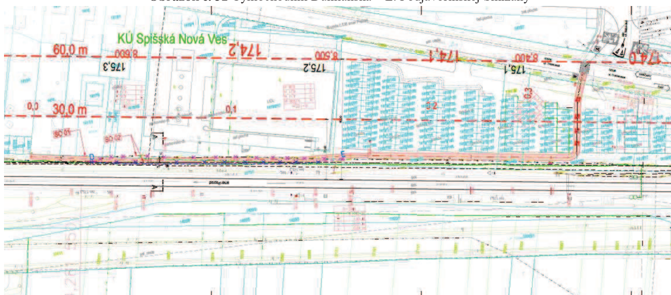
Obrázok č. 32 Cyklochodník Duklianska – E. Podjavorinskej Smižany
