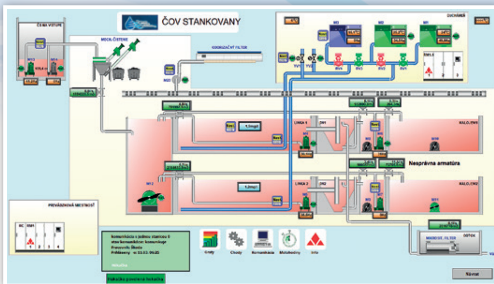
Dispečingový systém – Snímanie chodu ČOV Rojkov
