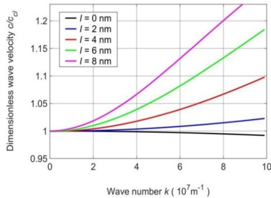
Figure 1. Bezrozmerná rýchlosť fázovej vlny c/c_d verzus vlnové číslo k pre f = 5 V a rôzne hodnoty parametrov dĺžkovej stupnice mikrotuhosti.
