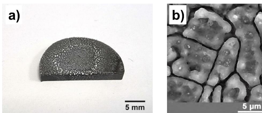
Obr. 1: a) povrch kompozitu B_4C s 5 hm.% SiC vlákien po vystavení kyslíkovo-acetylenovému plameňu pri teplote 1800^\circ C ; (b) SEM snímka povrchu B_4C -SiC kompozitu po laserovej ablácii pri teplote prevyšujúcej 10\,000\,K .
