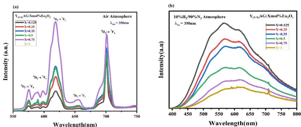
Obr. Fotoluminiscenčné emisné spektrá mikrogulôčiek YAG:Eu v rôznych koncentráciách a) pred redukciou, b) po redukcii v 10% H 2 /N 2
