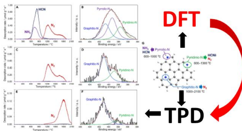
Obr. 1. Prípadová štúdia aplikácie metód TPD a DFT pre grafény s obsahom rôzneho typu dusíka. TPD profily a \text{N}1s XPS spektrá uhlíkového materiálu na báze porfyrínu.
