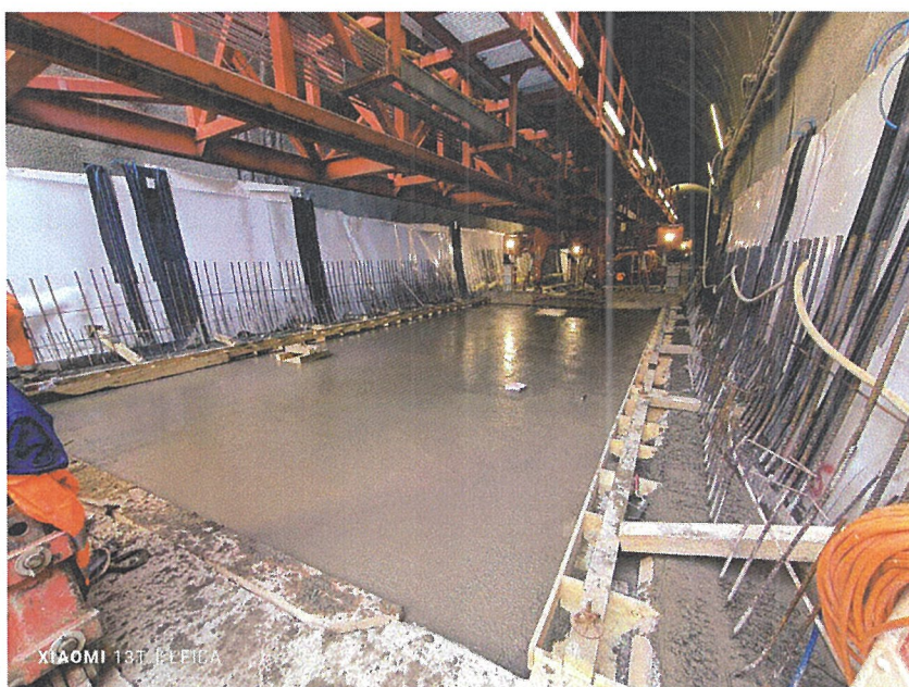
Tunnel Wendlingen
