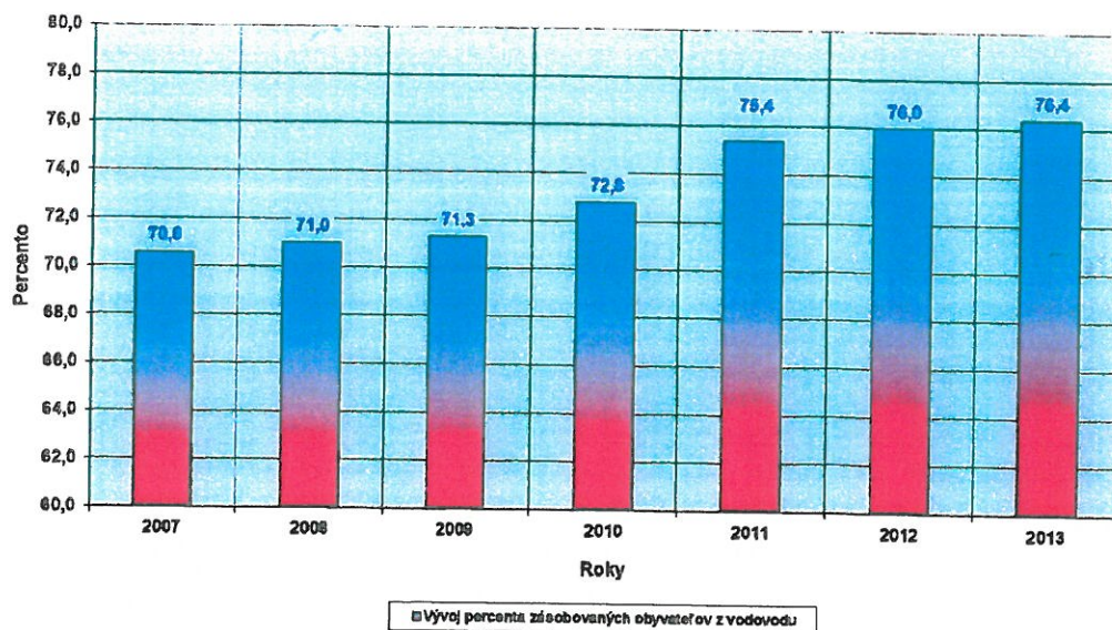
Vývoj percenta zásobovaných obyvateľov z vodovodu
