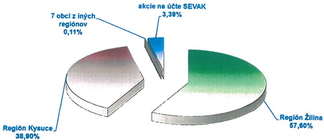
Percentuálny podiel na základnom imaní SEVAK, a.s. podľa regiónov v roku 2013
