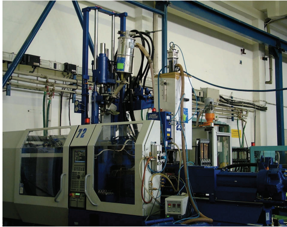
Vstrekovací lis DEMAG 150/500/610h/310/V - dvojkomponentný (dve vstrekovacie jednotky)
