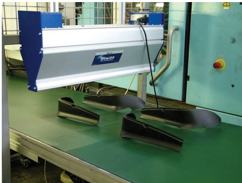
Ionizačná jednotka, ktorá odstráni znečistenie a prašnosť plastových dielcov
