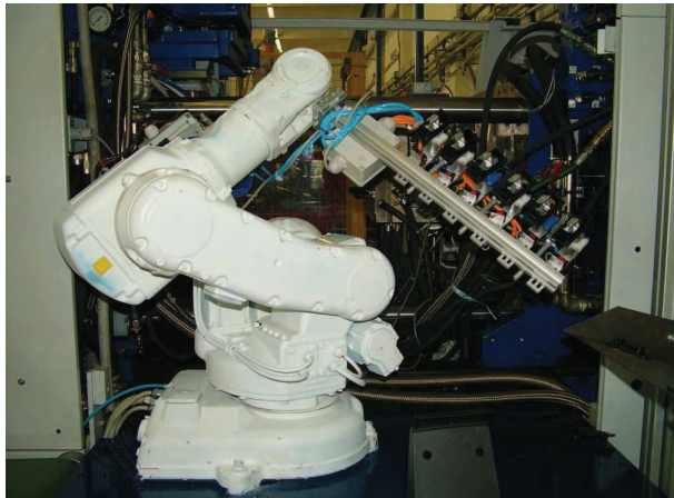
Šesťosí robot
