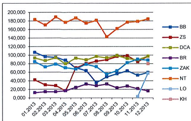
G2 – Mesačná výroba elektriny po zdrojoch v roku 2013 (v MWh)
