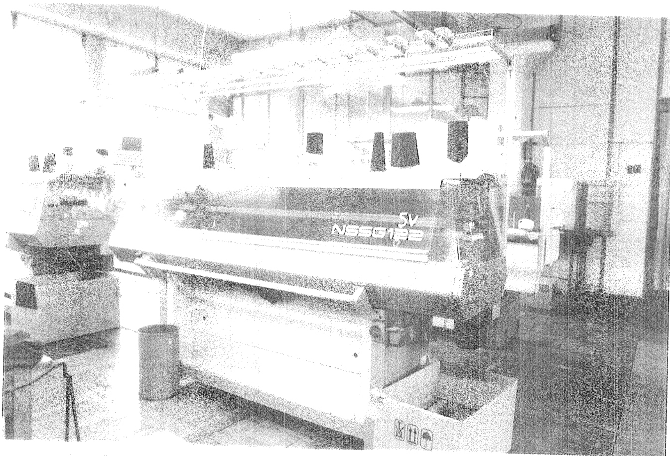
Plochý elektronicky riadený pletací stroj Shima Seiki NewSSG 122 SV 14G
