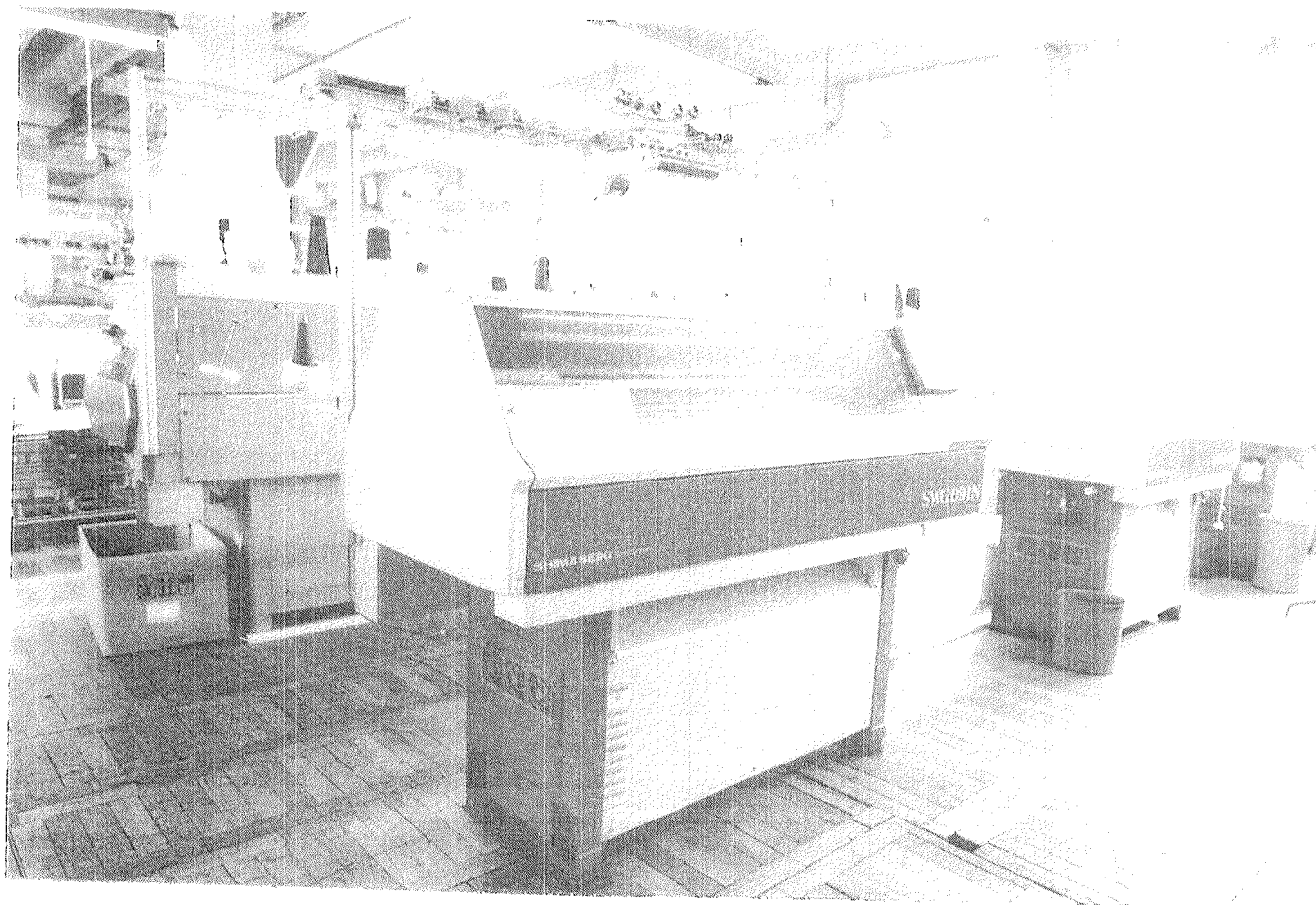
Elektronicky pletací stroj rukavicový automat Shima Seiki Swg 091 7gg
