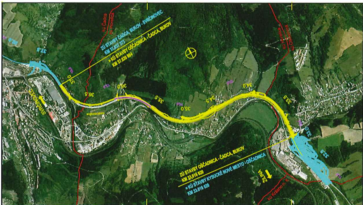
Obr. č. 14 Prehľadná situácia diaľnice
