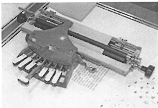
Obrázok č. 8: Stroj na písanie Braillovho písma
