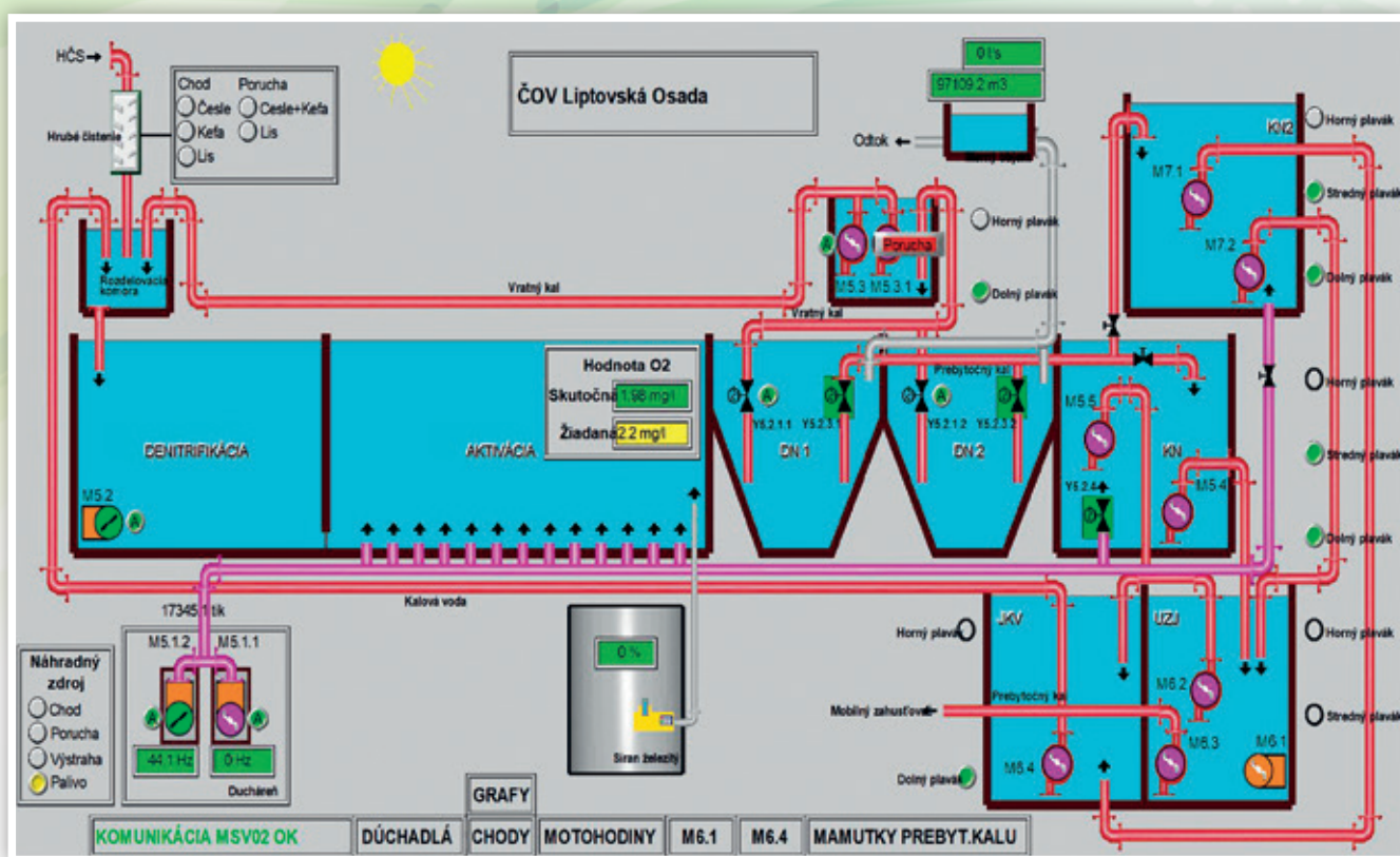
Dispečingový systém – Bloková schéma ČOV Liptovská Osada
