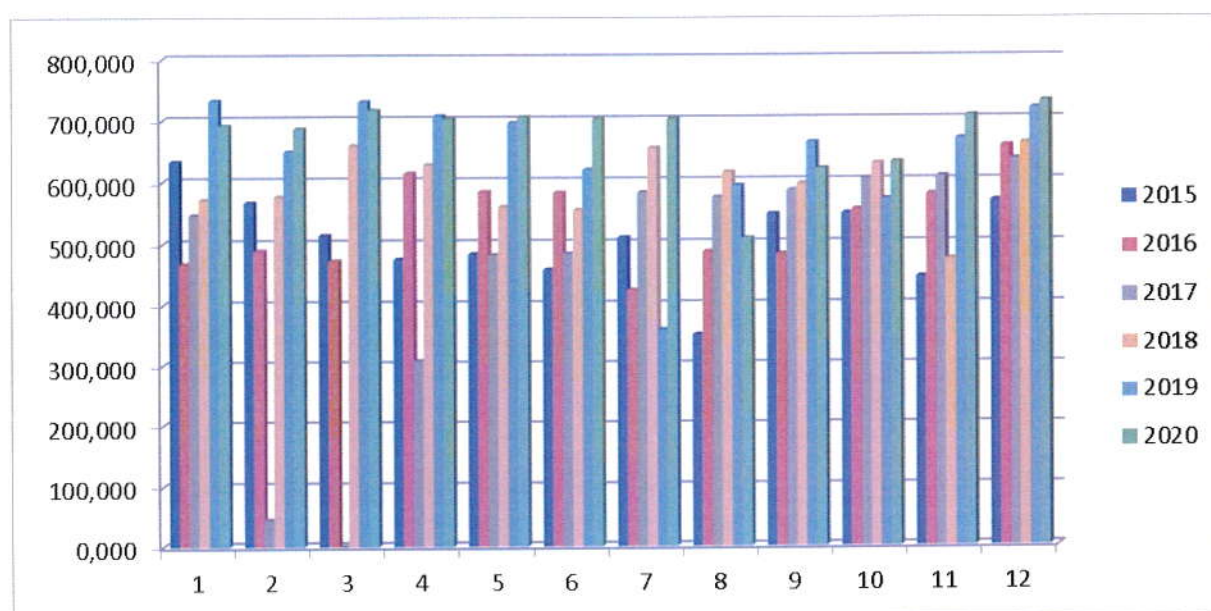
Graf č. 9 Vývoj výroby elektrickej energie na prevádzke č.1 v rokoch 2016 – 2020 po mesiacoch
