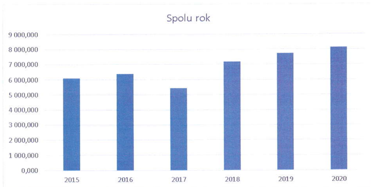
Graf č. 8 Vývoj výroby elektrickej energie na prevádzke č.1 v rokoch 2016 – 2020
