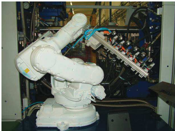
Šesťosí robot
